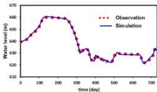
شکل ۳- مقایسه تراز سطح آب مشاهده‌ای و شبیه‌سازی شده در مخزن سد سیمره
