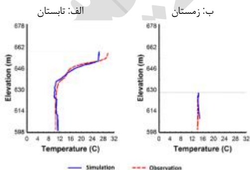
شکل ۴- مقایسه توزیع دمای مشاهده‌ای و شبیه‌سازی شده در مخزن سد سیمره
